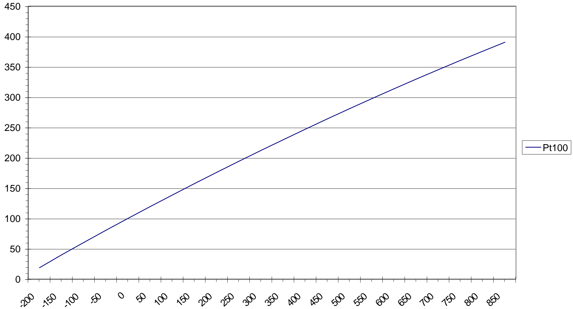
Widerstandswerte Pt100 Sensoren
